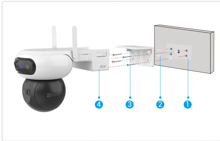
圖 2 壁掛式安裝
